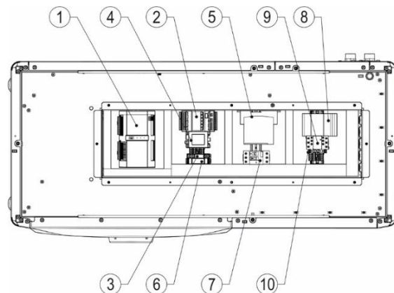
Rysunek 3. Sterownik obiegu chłodniczego w jednostce zewnętrznej. 1-sterownik obiegu chłodniczego; 2-sterownik zaworu rozprężnego; 3-przełącznik; 4-transformator napięcia; 5-soft-start; 6-czujnik kontroli i zaniku faz; 7-wyłącznik silnikowy sprężarki; 8-licznik energii; 9-stycznik grzałki; 10-bezpiecznik.
